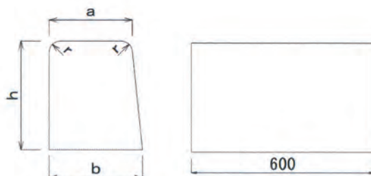
歩車道境界ブロック (両面7型)
