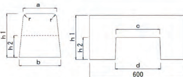
歩車道境界ブロック (水抜き 8型)
