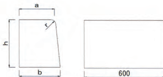
歩車道境界ブロック (片面 基本)
