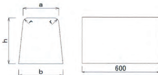
歩車道境界ブロック (両面 8 型)
