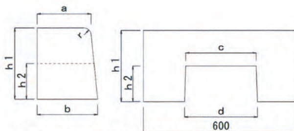
歩車道境界ブロック (水抜き 基本)
