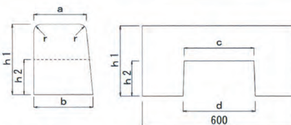
歩車道境界ブロック (水抜き 7型)
